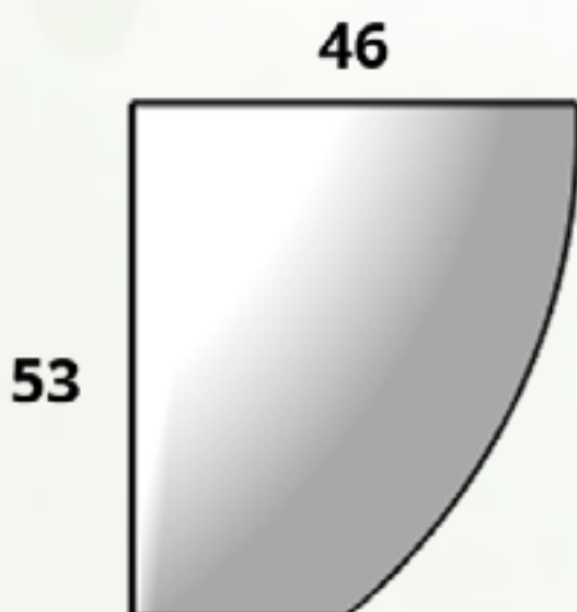
CÓDIGO VENECIA PARED 04 Diám. Boca x Ancho x Altura 110 cm x 46 cm x 53 cm
