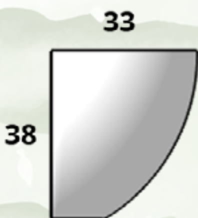
CÓDIGO VENECIA PARED 03 Diám. Boca x Ancho x Altura 79 cm x 33 cm x 38 cm
