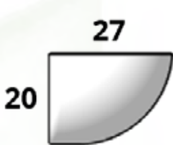
CÓDIGO VENECIA PARED 02 Diám. Boca x Ancho x Altura 40 cm x 27 cm x 20 cm
