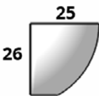
CÓDIGO VENECIA PARED 05 Diám. Boca x Ancho x Altura 56 cm x 25 cm x 26 cm
